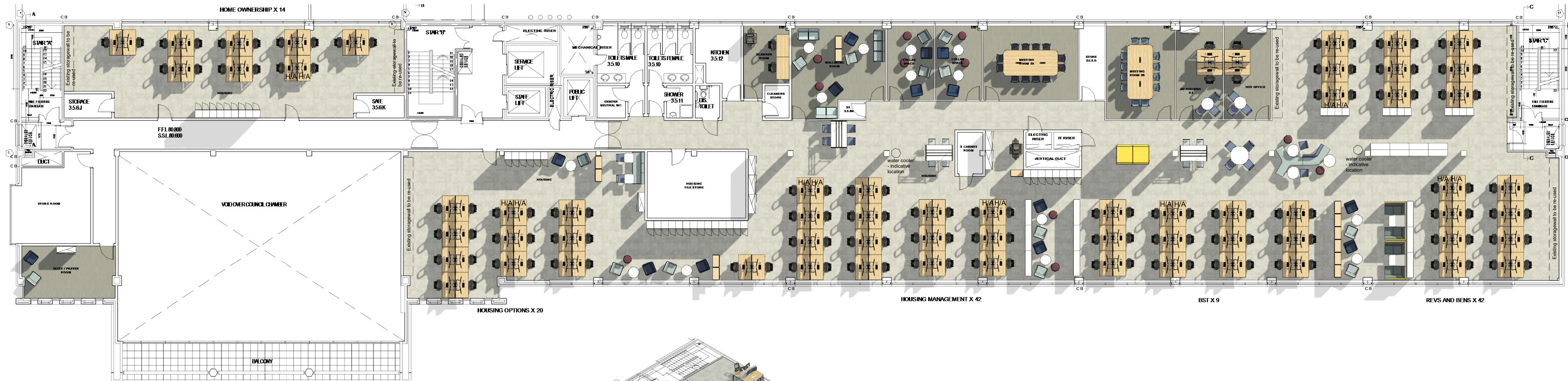
1 Level 02 1 : 125
